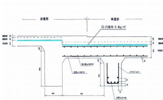
施工概要図
