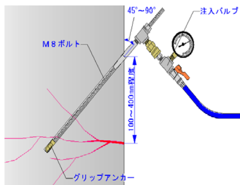
注入工法概要図
