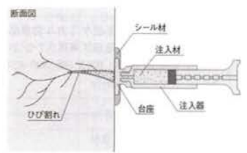
図 注入工法概要図(断面図)
